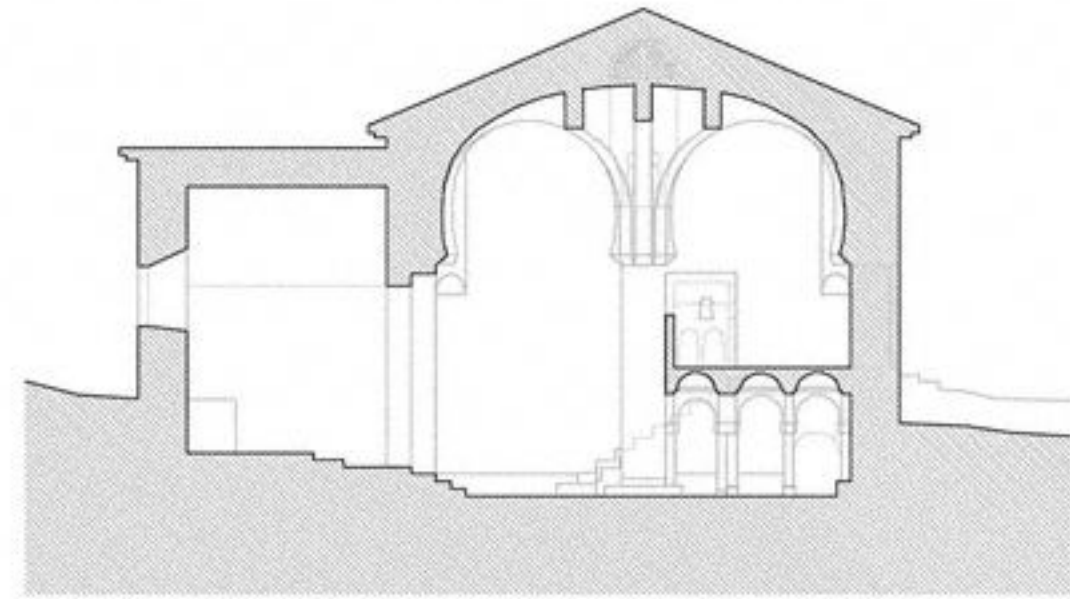
SECCIÓN L-L''
