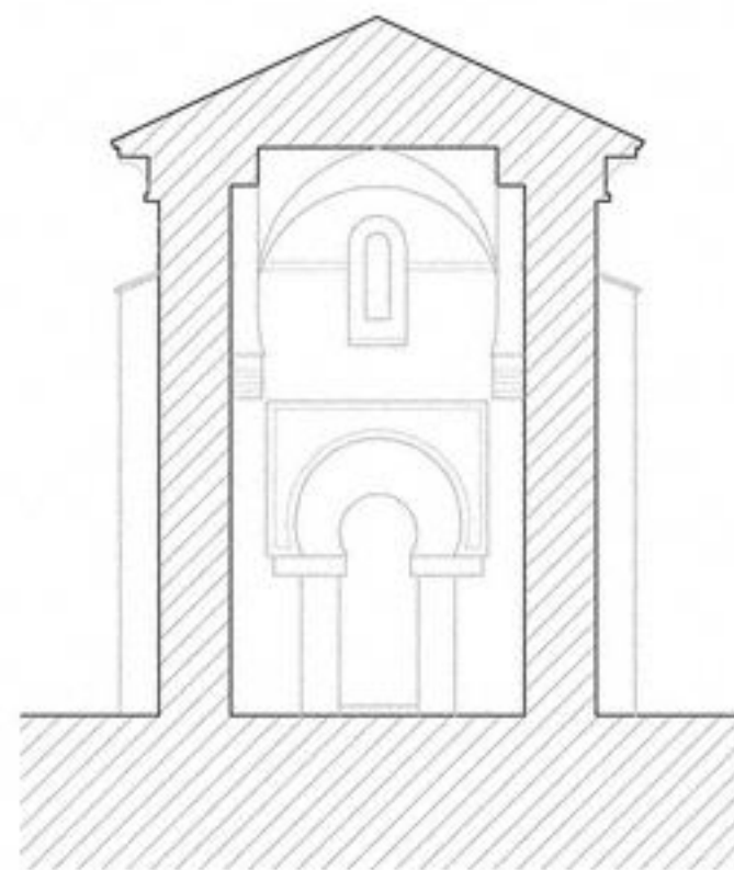
SECCIÓN TRASVERSAL E 1:100
