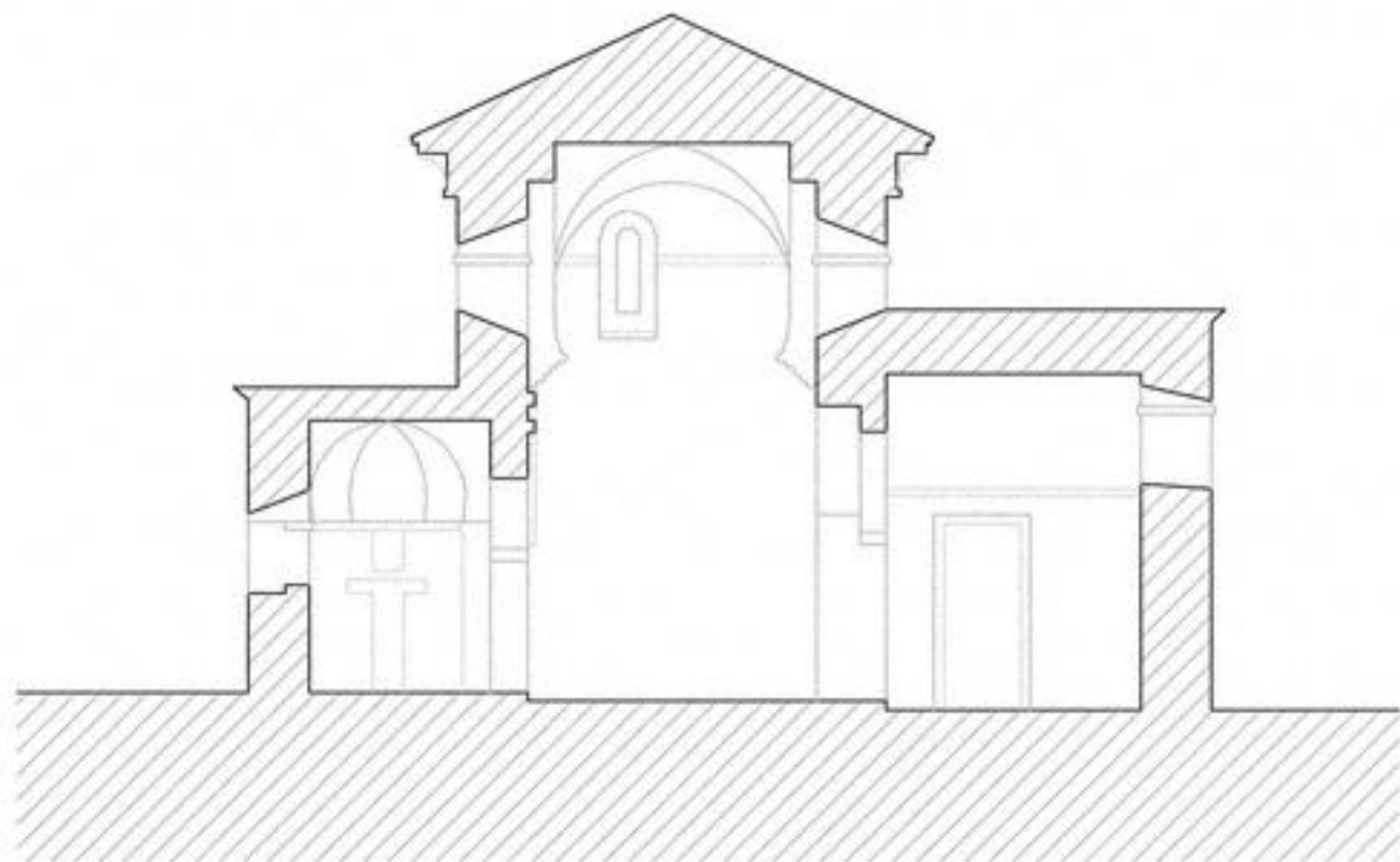
SECCIÓN LONGITUDINAL E 1:100
