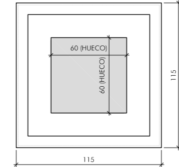
L3 LUCERNARIO SALA DE EXPOSICIONES PEQUEÑA Y ASEOS VIDRIO DOBLE: LAMINAR (8+8 mm) SISTEMA DE OSCURECIMIENTO MECÁNICO 14 UDS.
