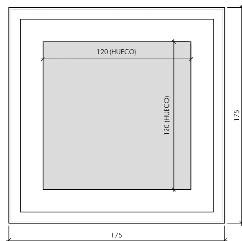
L4 LUCERNARIO TALLER DE ARTISTAS Y SALA DE REUNIONES VIDRIO DOBLE: LAMINAR (8+8 mm) SISTEMA DE OSCURECIMIENTO MECÁNICO 2 UDS.
