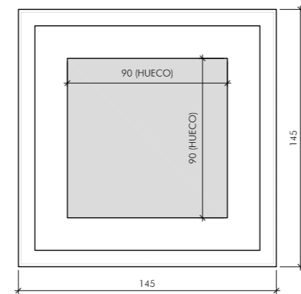
L2 LUCERNARIO SALA EXPOSICIONES MEDIANA VIDRIO DOBLE: LAMINAR (8+8 mm) SISTEMA DE OSCURECIMIENTO MECÁNICO 4 UDS.
